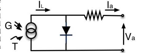
Fig. 7. Solar PV circuit.
